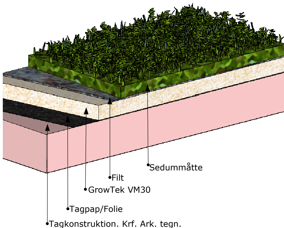
Principopbygning GrowTek VM30 sedum tag
