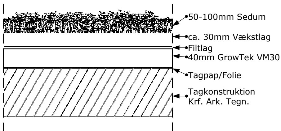
Principsnit GrowTek VM30 sedum tag
