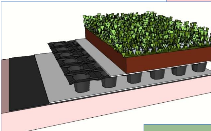
VMP25 Opbygningshøjde: 50mm Maks. vægt: 38kg/kvm Vandtilbageholdelse: 27ltr/kvm
