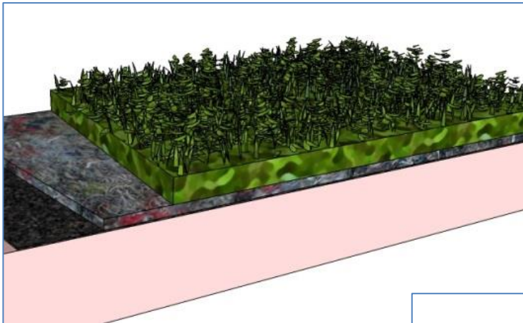
VMF12 Opbygningshøjde: 50mm Maks. vægt: 39kg/kvm Vandtilbageholdelse: 25ltr/kvm
