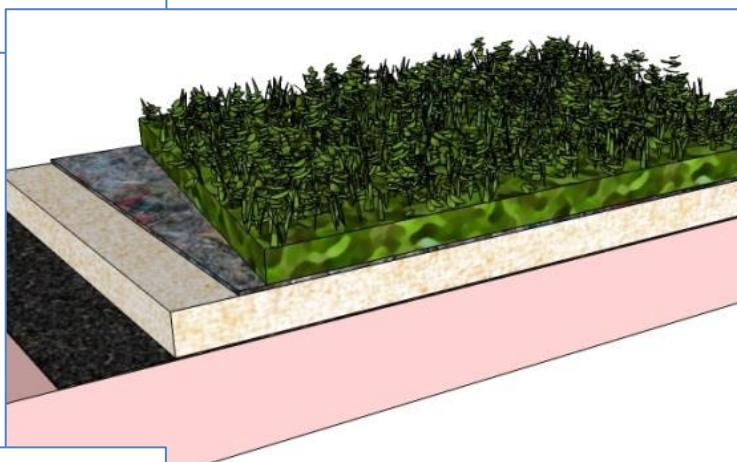
VM30 Opbygningshøjde: 70mm Maks. vægt: 52kg/kvm Vandtilbageholdelse: 45ltr/kvm
