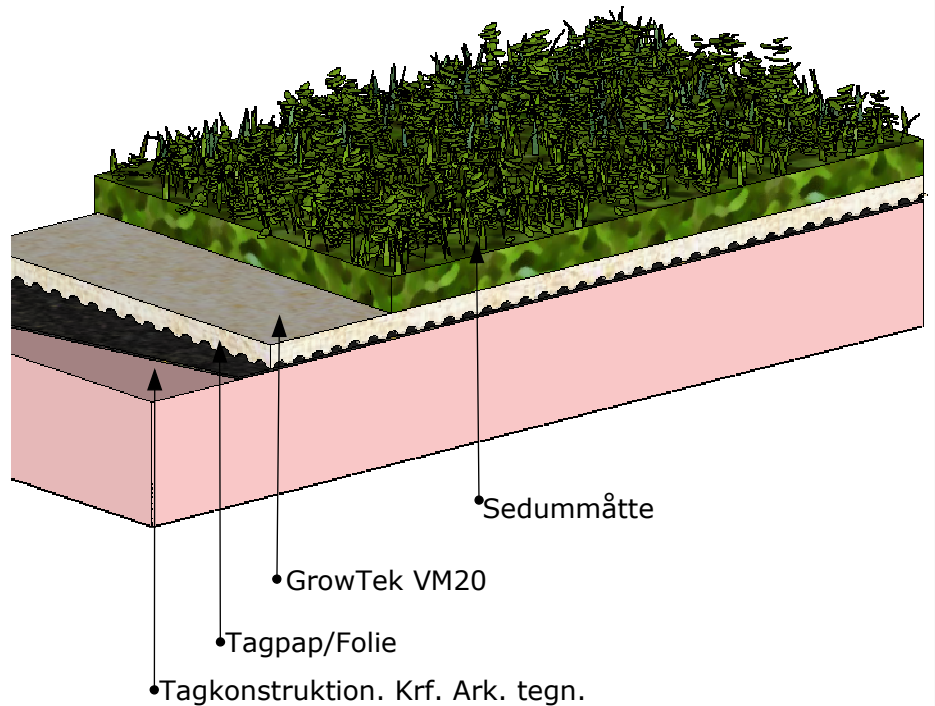
Principopbygning GrowTek VM20 sedum tag
