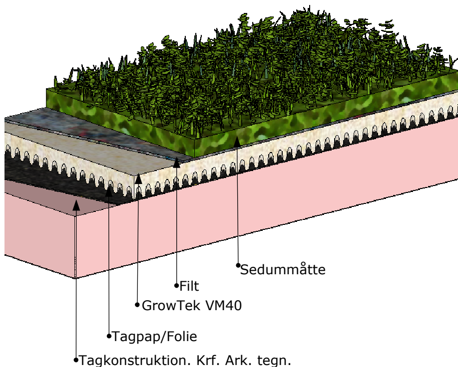
Principopbygning GrowTek VM40 sedum tag
