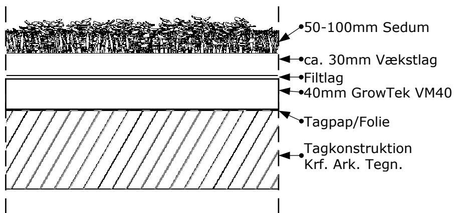
Principsnit GrowTek VM40 sedum tag
