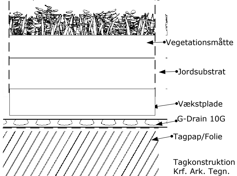
Principsnit i Growtek VMH40 Grønt Tag.
