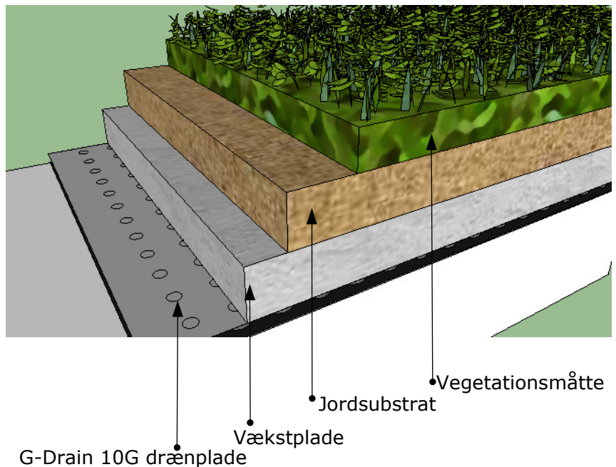
Principsnit i Growtek VMH40 Grønt Tag.
